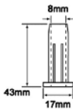
Gniazdo plastikowe
