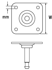
Płyta montażowa
