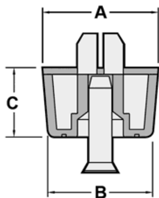
PRZED MONTAŻEM BEFORE INSERTION
