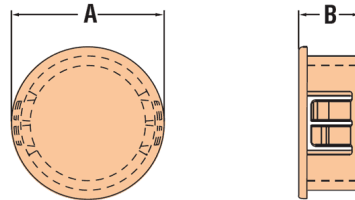
Wiele stopni blokujących Multiple panel thickness design
