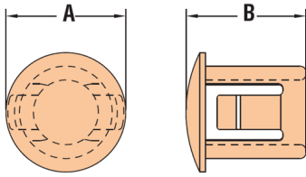
Pojedynczy stopień blokujący Single panel thickness design
