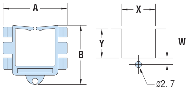
Wycięcie krawędziowe Edge slot
