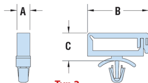
Typ 2 Type 2
