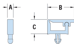
Typ 1 Type 1
