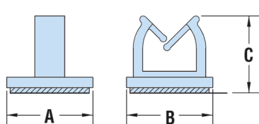
Typ 1 Type 1
