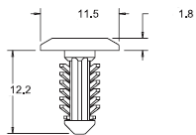
BPF-F2495
